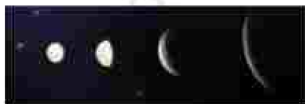
Fig. 17.20 : Phases of Venus
